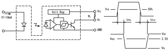
伝搬時間測定条件 / Measurement of propagation time
