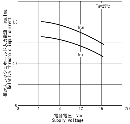
■ 相対スレッシユホールド入力電流/ 電源電圧特性 I_{FLH}, I_{FHL}/V_{CC}
