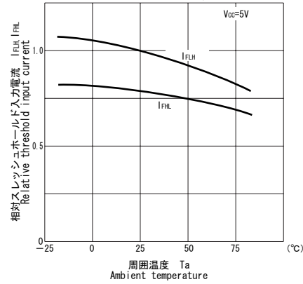
■ 相対スレッシユホールド入力電流/ 周囲温度特性 I_{FLH}, I_{FHL}/T_a
