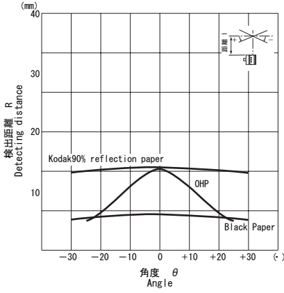
■ 検出距離／角度特性 R/θ
