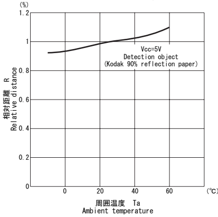
■ 検出距離／周囲温度特性 R/Ta
