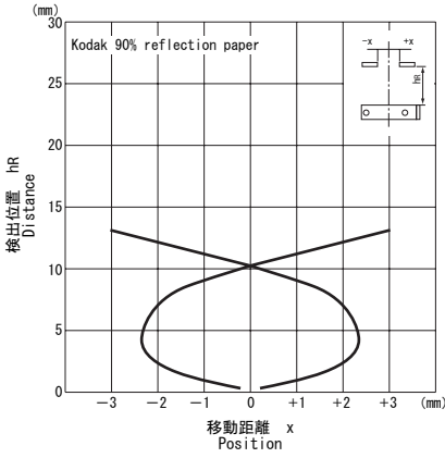
■ 検出位置／移動距離特性 hR/x
