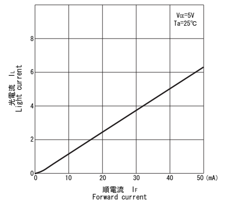
■光電流/順電流特性 I_L/I_F
